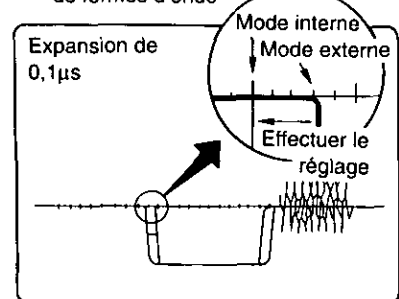
■ Forme d'onde sur le moniteur de formes d'onde
