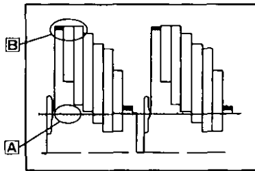
Forme d'onde sur le moniteur de formes d'onde
